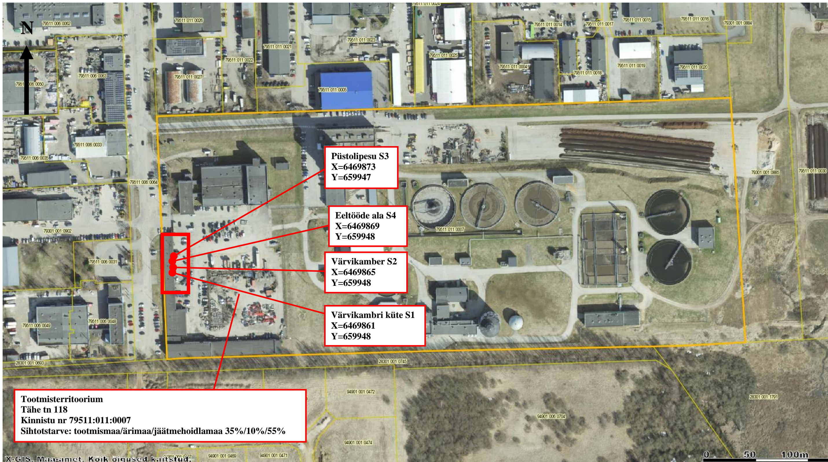
Käitise asendiplaan, tootmisterritoriumi piir ja heiteallikad.
