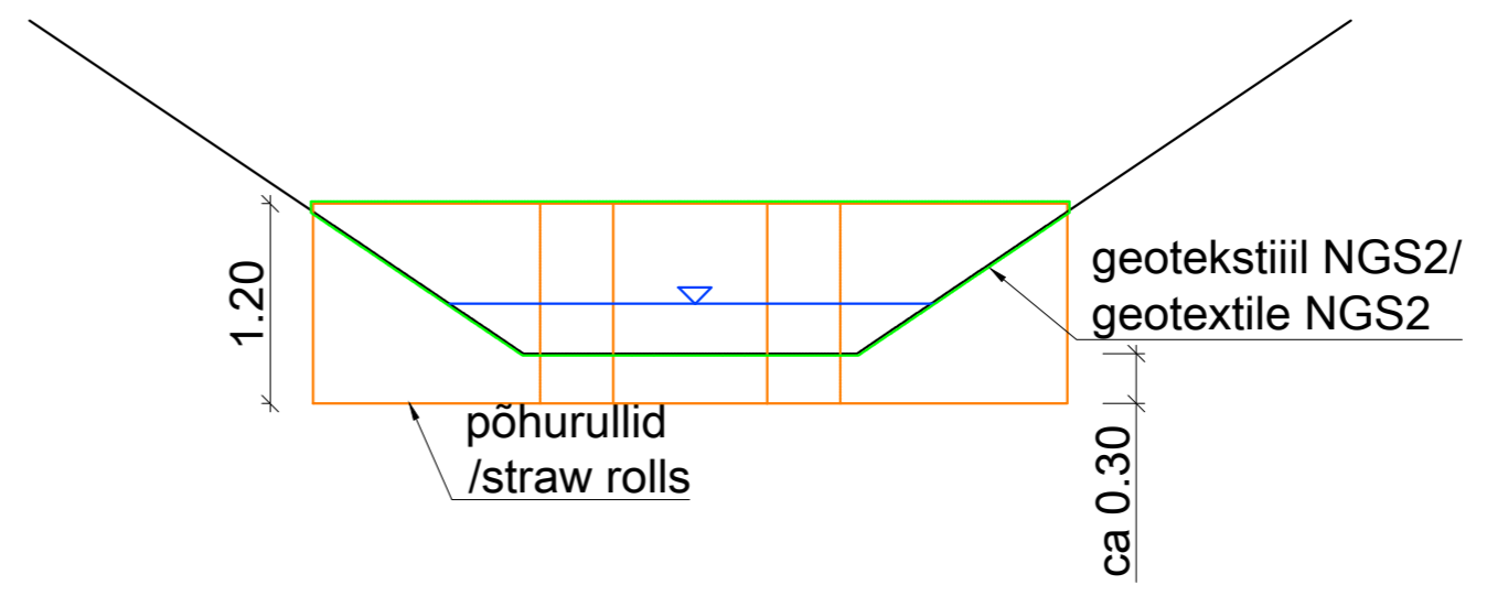
Settekraani ristlõige / Sediment screen cross-section
