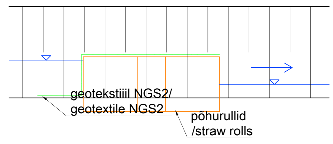
Settekraani pikilõige / Sediment screen longitudinal section
