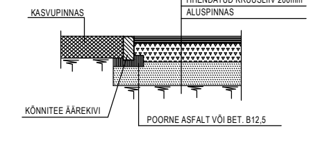
LÕIGE 4-4
