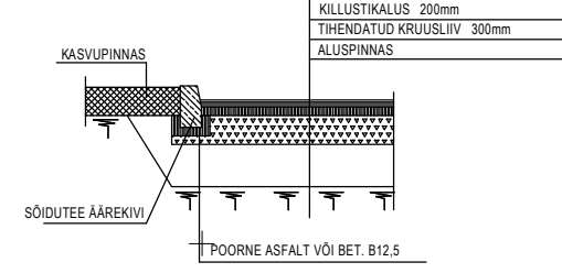
LÕIGE 1-1
