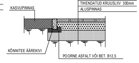
LÕIGE 3-3
