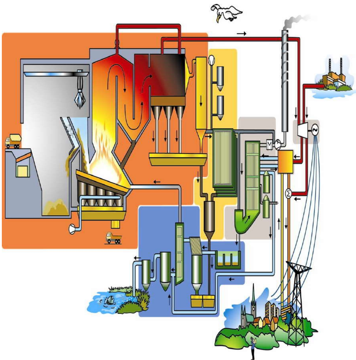
Figur 3 Processbild Gärstadverket förbränningslinje 4.
