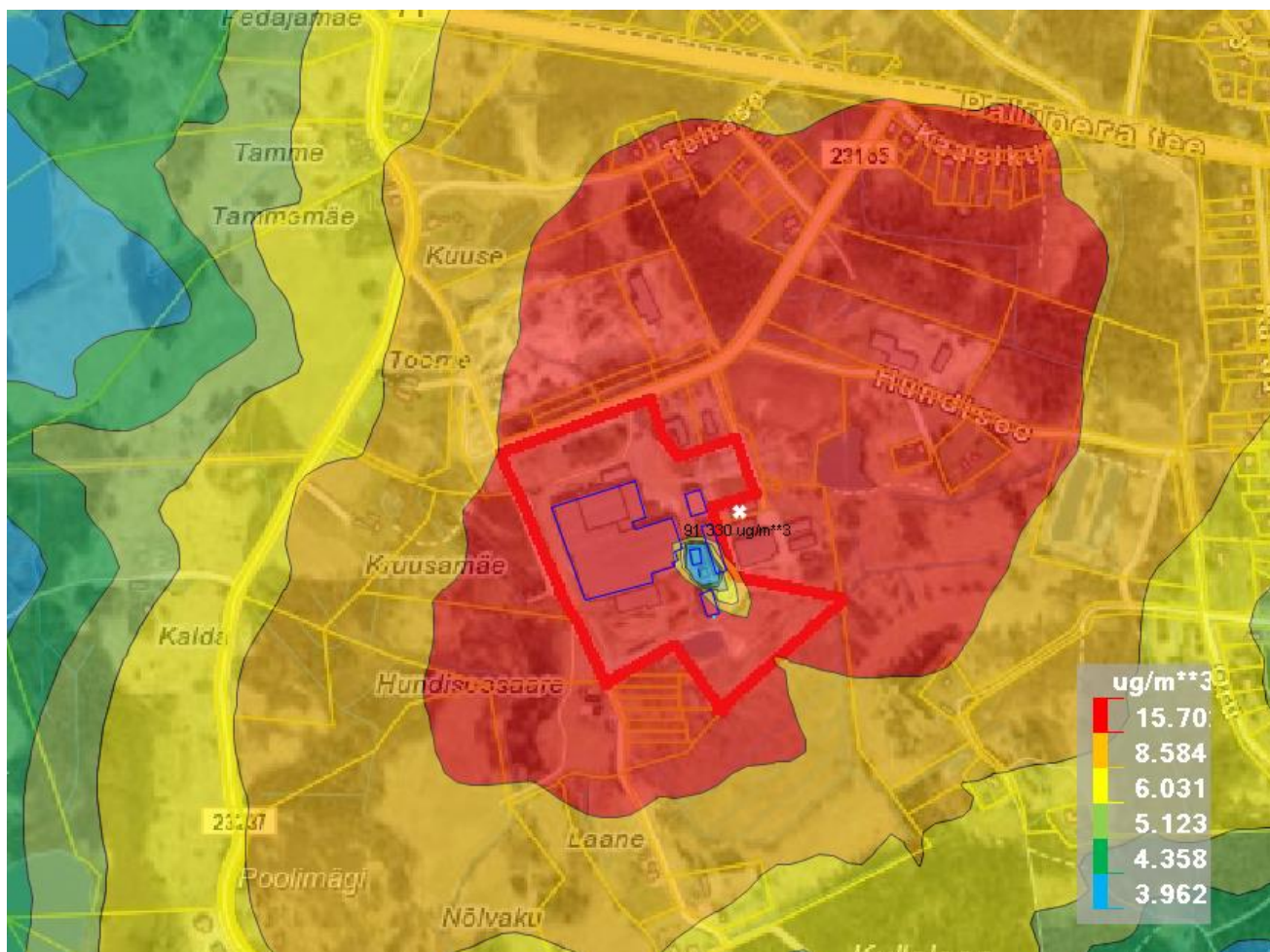
Joonis L8.2. Väeveldioksiidi hajumise 24-tunni keskmised maapinnalähedased koosmõju kontsentratsioonid vastavalt lisatud värviskaalale (reservkatlamaja korsten 1). Maksimaalne kontsentratsioon 91,330 µg/m³ (asukoht tähistatud tärniga). \text{ÖPV}_{24}=125\mu\text{g}/\text{m}^3
