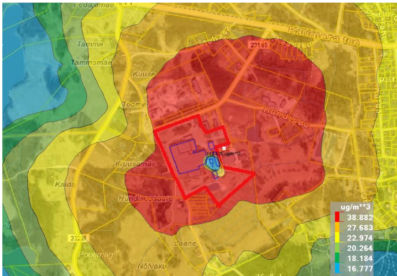
Joonis L8.1. Väeveldioksiidi hajumise tunnikeskmsed maapinnalähedased koosmõju kontsentratsioonid vastavalt lisatud värviskaalale (reservkatlamaja korsten). Maksimaalne kontsentratsioon 113,626 \mu\text{g}/\text{m}^3 (asukoht tähistatud tärniga). \text{ÖPV}_1=350 \mu\text{g}/\text{m}^3
